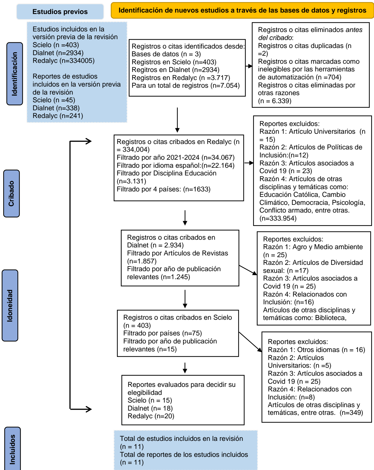
Figura 1. Diagrama PRISMA
